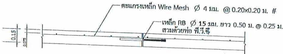
EXPANSION JOINT(ทุกระยะ 100.00 เมตร)
