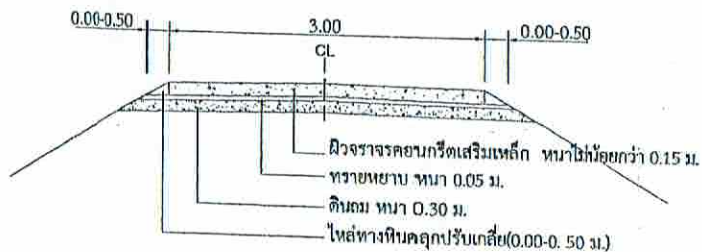
รูปตัดถนนผิวจราจรคอนกรีตเสริมเหล็ก
